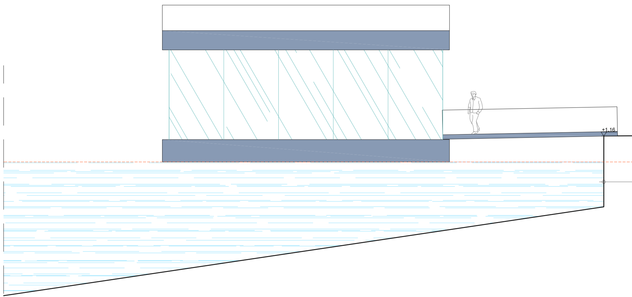
OBALA VRSARA, PRESJEK mjerilo 1:100
